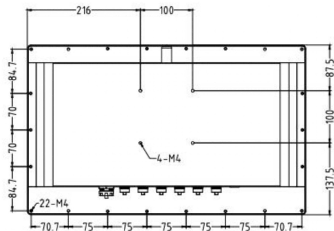
背视图
