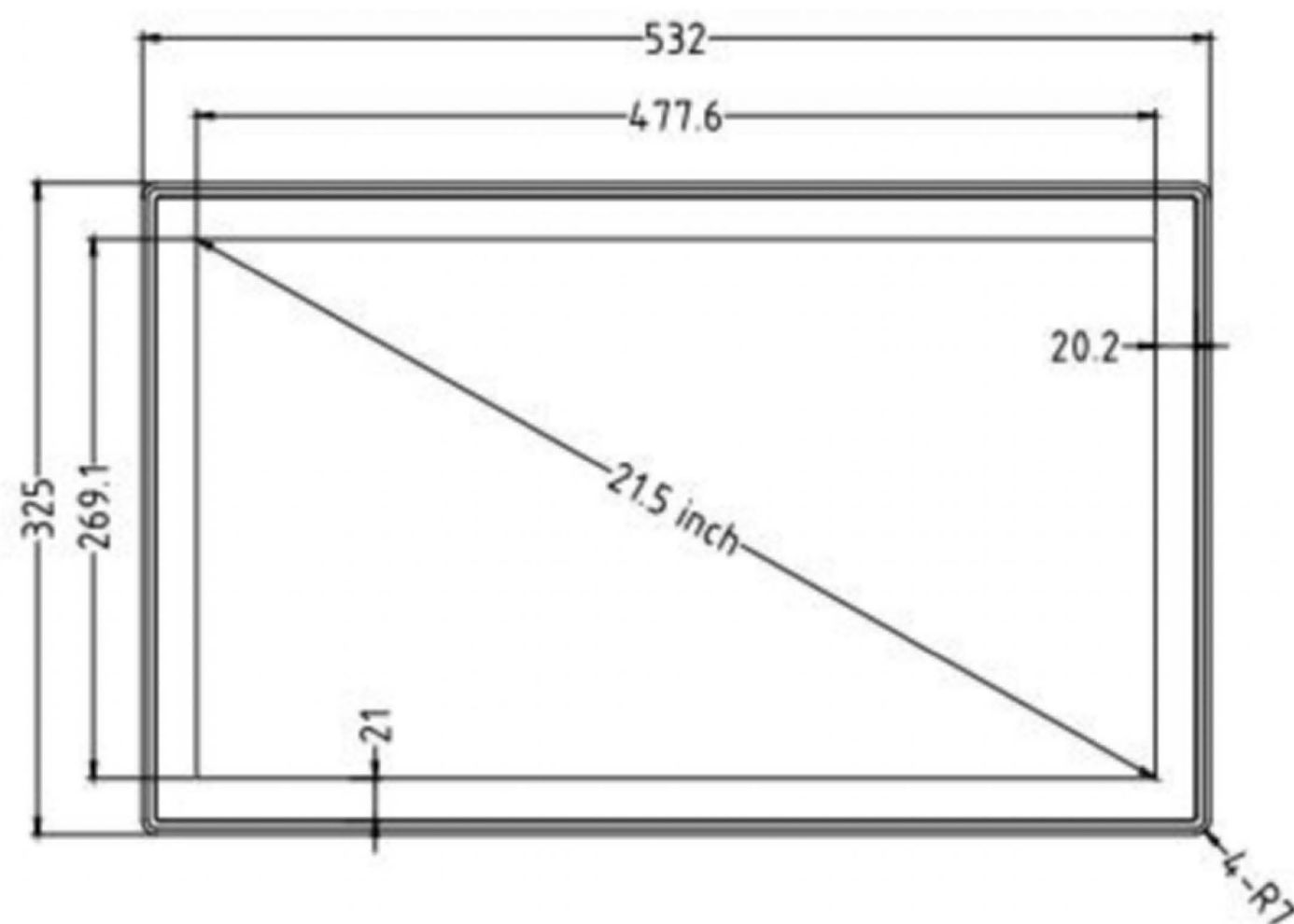
正视图
